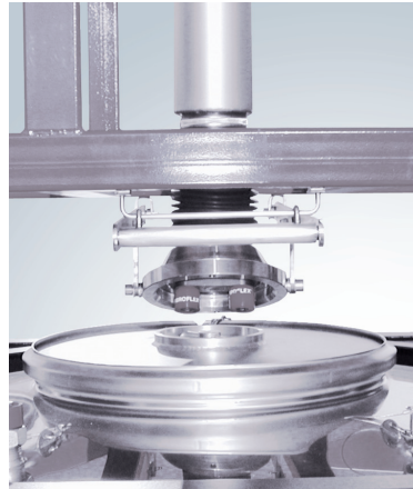
Симплексное соединение привода к устройству для перемешивания.
